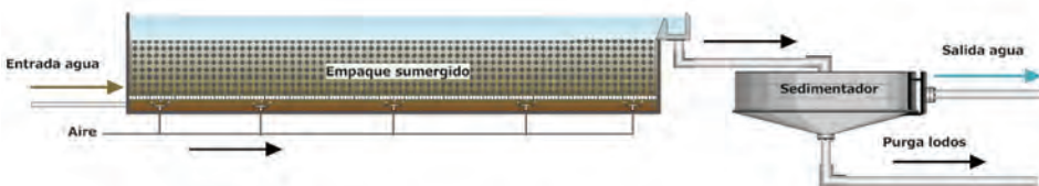
Figura 1.9. Procesos aerobios para el tratamiento de aguas residuales.
