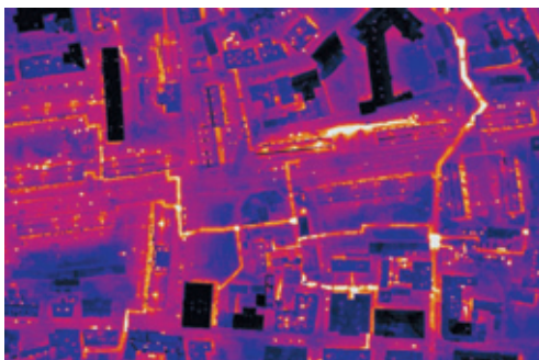
Imagen 23. Termografía aplicada a District Heating. Fuente: Horuslab .
