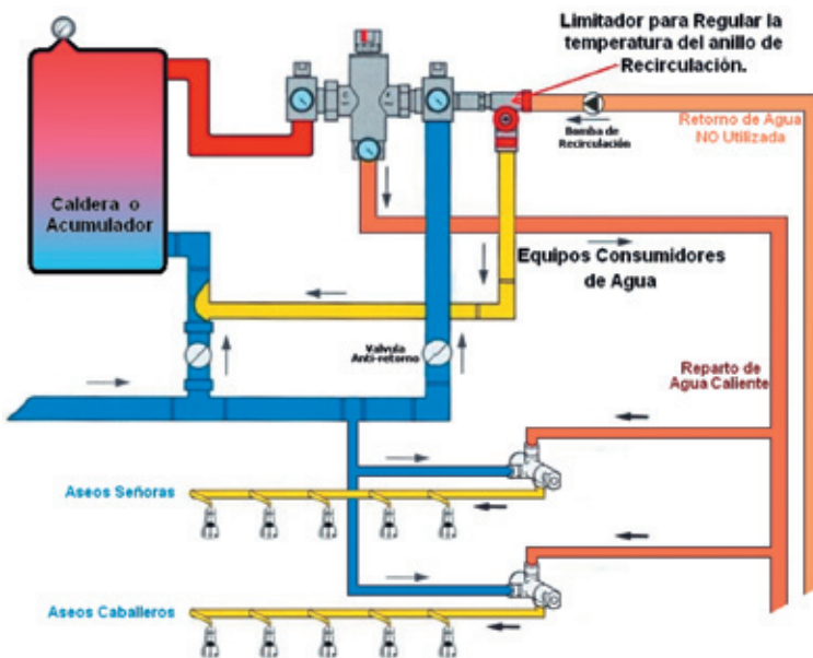
Figura 1. Circuito optimizado termostático de agua caliente con anillo de recirculación
