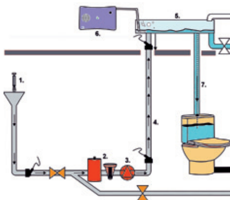
Figura 5. Módulo para la reutilización de aguas grises en cuarto húmedo. (Fuente: Ecoplay – Ecohoe).
