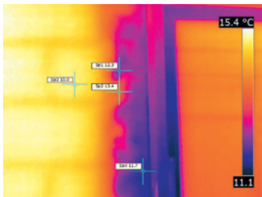
Imagen 3. La capilaridad del agua hace que esta tenga un patrón característico. La huella térmica del agua es casi siempre difusa y muy diferenciable de la de la infiltración de aire, más rectilínea.
