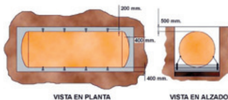
Foto 9. Instalación de un depósito enterrado.
