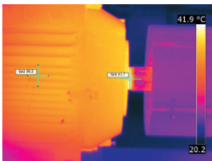
Imagen 11. Las bombas circuladoras de agua se inspeccionaron para localizar posibles contactos eléctricos sobrecalentados, desequilibrios en los ejes o desgaste en los rodamientos y falta de bobinados.
