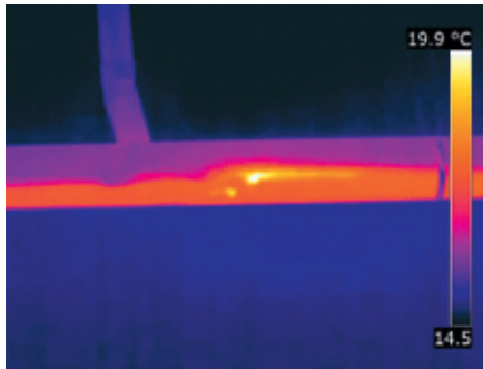
Imagen 16. Localización de un posible sedimento que no termina de ser arrastrado y al que habrá que observar en futuras inspecciones.
