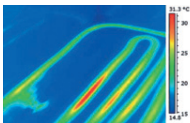
Imagen 19. Para la localización con total precisión el punto exacto de una fuga en una instalación de suelo radiante, evitando así tener que levantar el suelo por completo.
