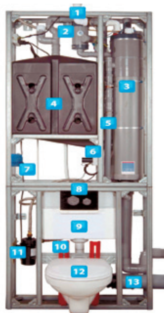
Figura 4. Módulo para la reutilización de aguas grises por ozonización. Fuente: Stella Energy, S.L. - In Tec Dolo.
