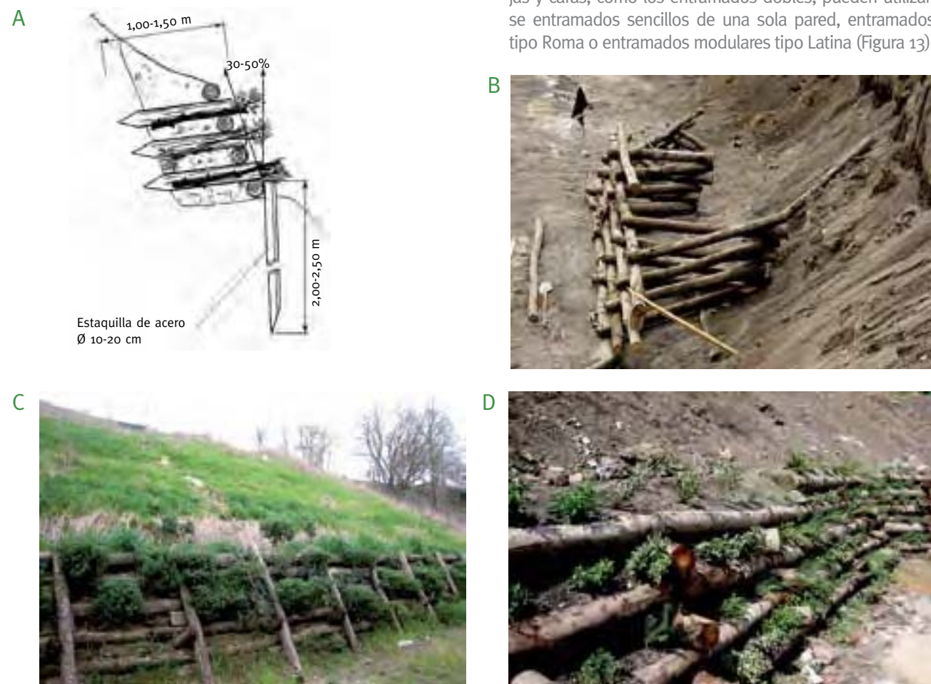
Figura 13. Entramado sencillo de una pared (A, tomado de Florineth 2004), entramado tipo 'Roma' (Paolo Cornellini, B), y entramado tipo 'Latina' (Paolo Cornellini y Sauli; 2005, C y D).
