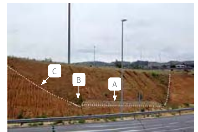
Figura 1. La presión constructiva sobre muchos territorios es tal que, como en el caso que muestra la fotografía, el trazado de una carretera anterior, relleno por materiales de escombrera, puede quedar incorporado, a modo de registro sedimentario, en el desmonte de una carretera más reciente. La línea blanca discontinua señala esta exposición singular. Sobre ella pueden identificarse un corte perpendicular de la plataforma de la carretera, el asfalto (A), las cunetas (B) y los antiguos desmontes (C) (Foto: F. Barbero).
