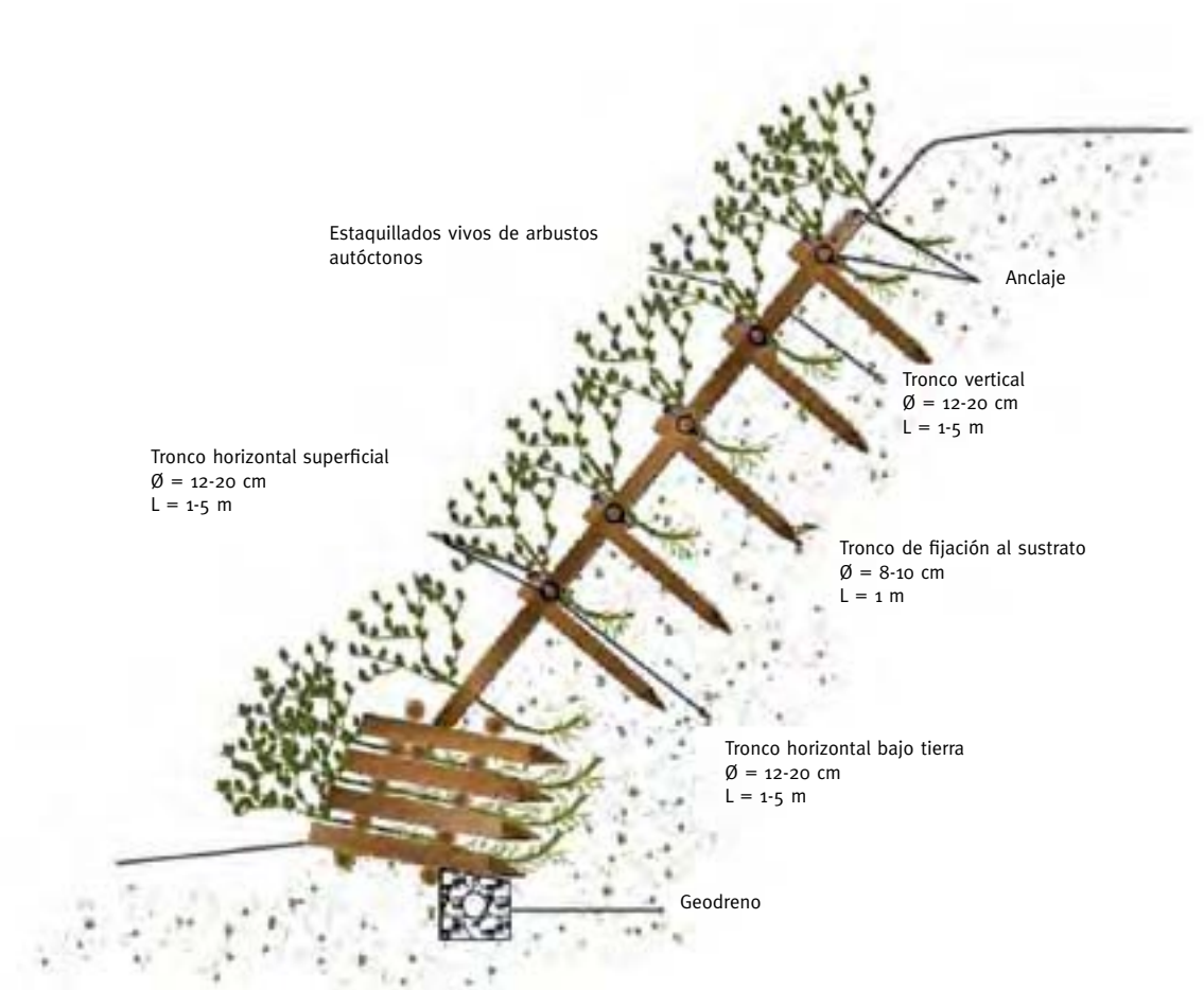
Figura 12. Entramado vivo doble combinado con un enrejado vivo y un drenaje para el soporte y consolidación de una pendiente (tomado de Martinho 2005).
