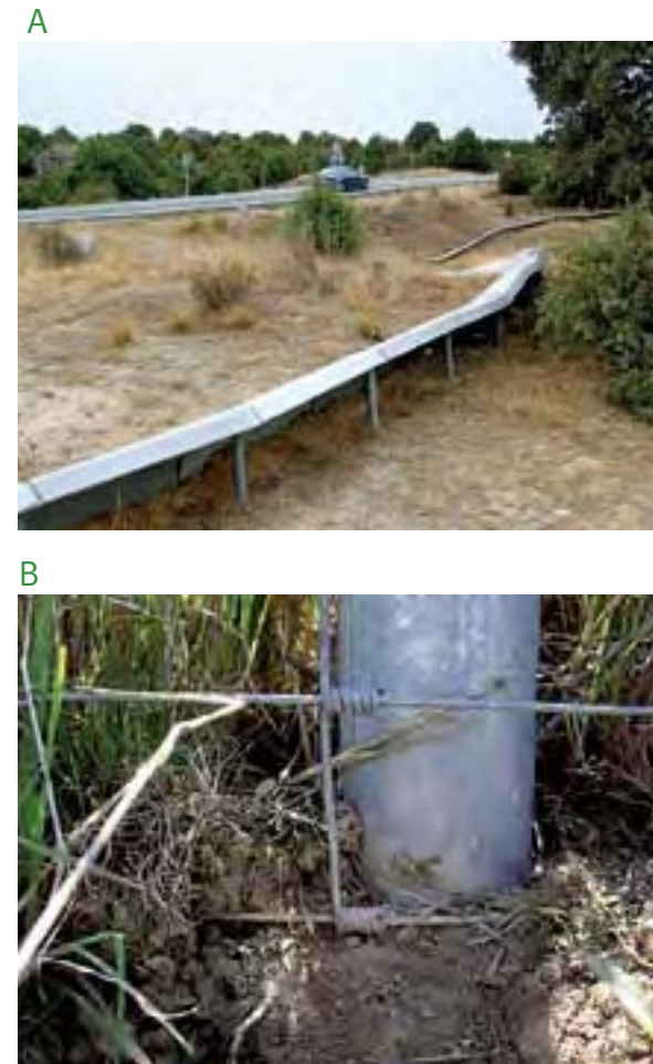
Figura 3. Ejemplos de buenas prácticas en cerramientos: vallado especial para evitar el acceso de anfibios a la calzada (A), ubicado en un tramo conflictivo por el paso estacional de anfibios en la carretera M-618 (Madrid), y detalle de vallado enterrado en la base (B) en la autopista AP-51 en la provincia de Ávila.
