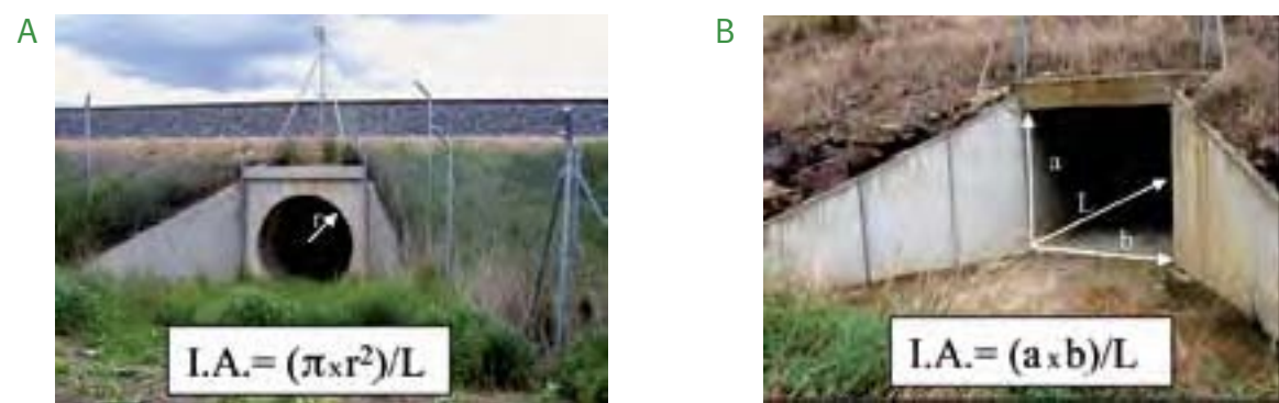
Figura 6. Ejemplos de cálculo del índice de apertura en dos drenajes de diferente sección: drenaje circular (izquierda) y drenaje adecuado (derecha).
