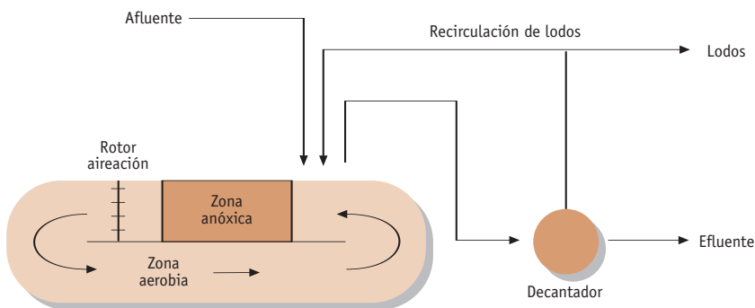
FIGURA 2.10 Canal de oxidación.
