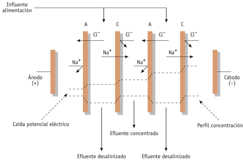
FIGURA 3.10 Equipo de electrodiálisis.
