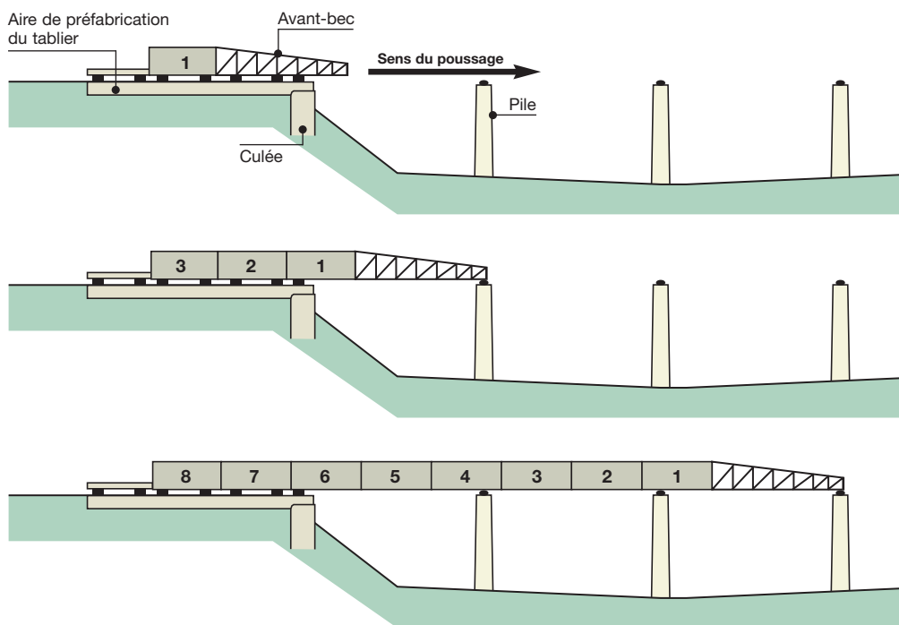
Figure n°1 : Construction par poussage
