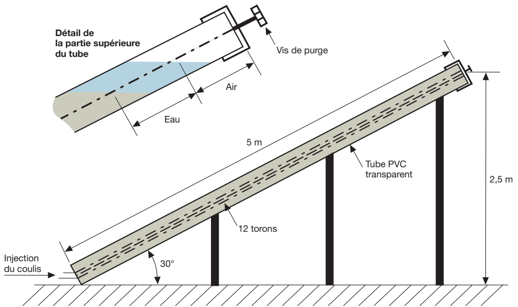
Figure n°6 : Dispositif d'essai de stabilité sur tube incliné
