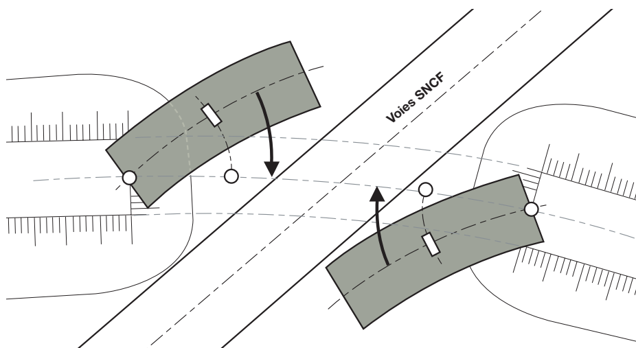
Figure n°2 : Construction par rotation
