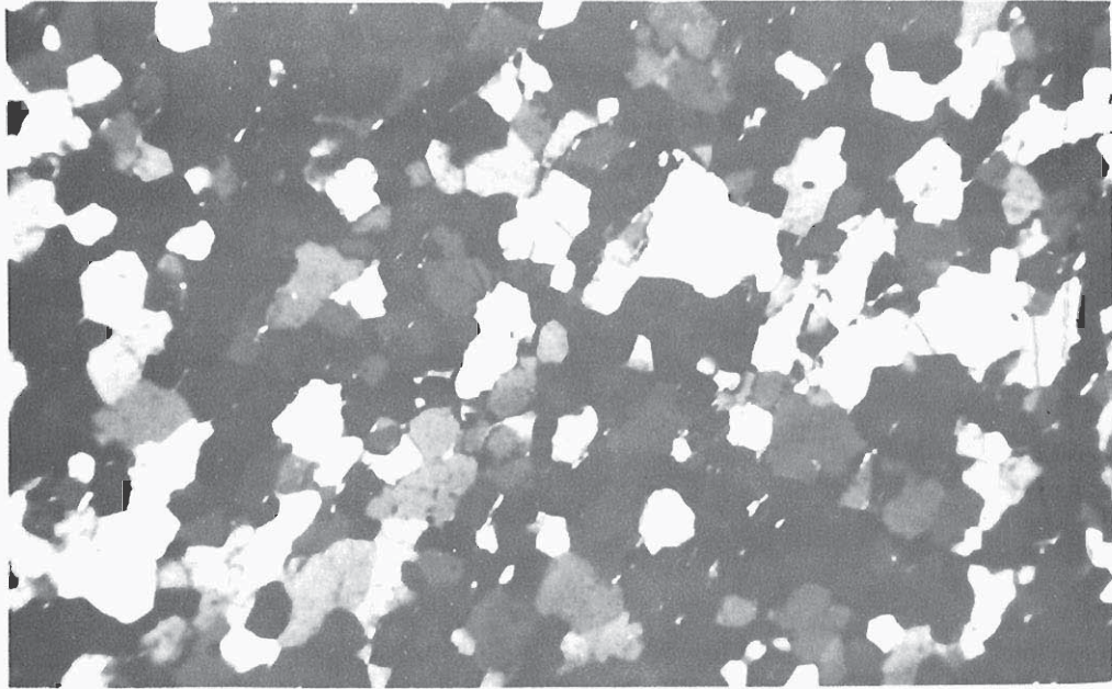
Foto 14.— Mosaico equigranular de cuarzo formando la típica textura granoblástica de una muestra de cuarcita armoricana (121b) (50 aumentos).
