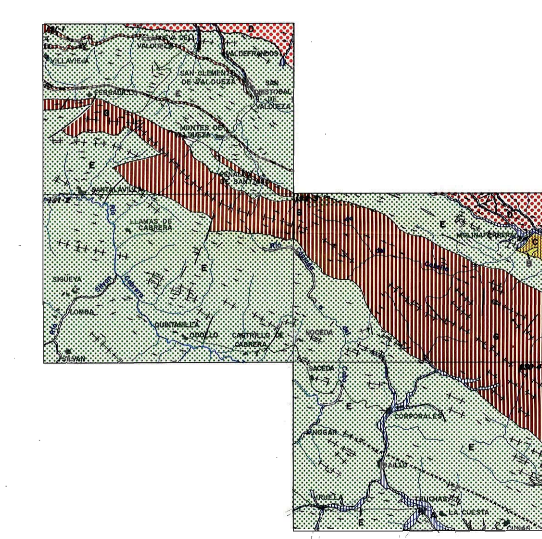
ESQUEMA MORFOLOGICO / ESCALA 1: 200.000
