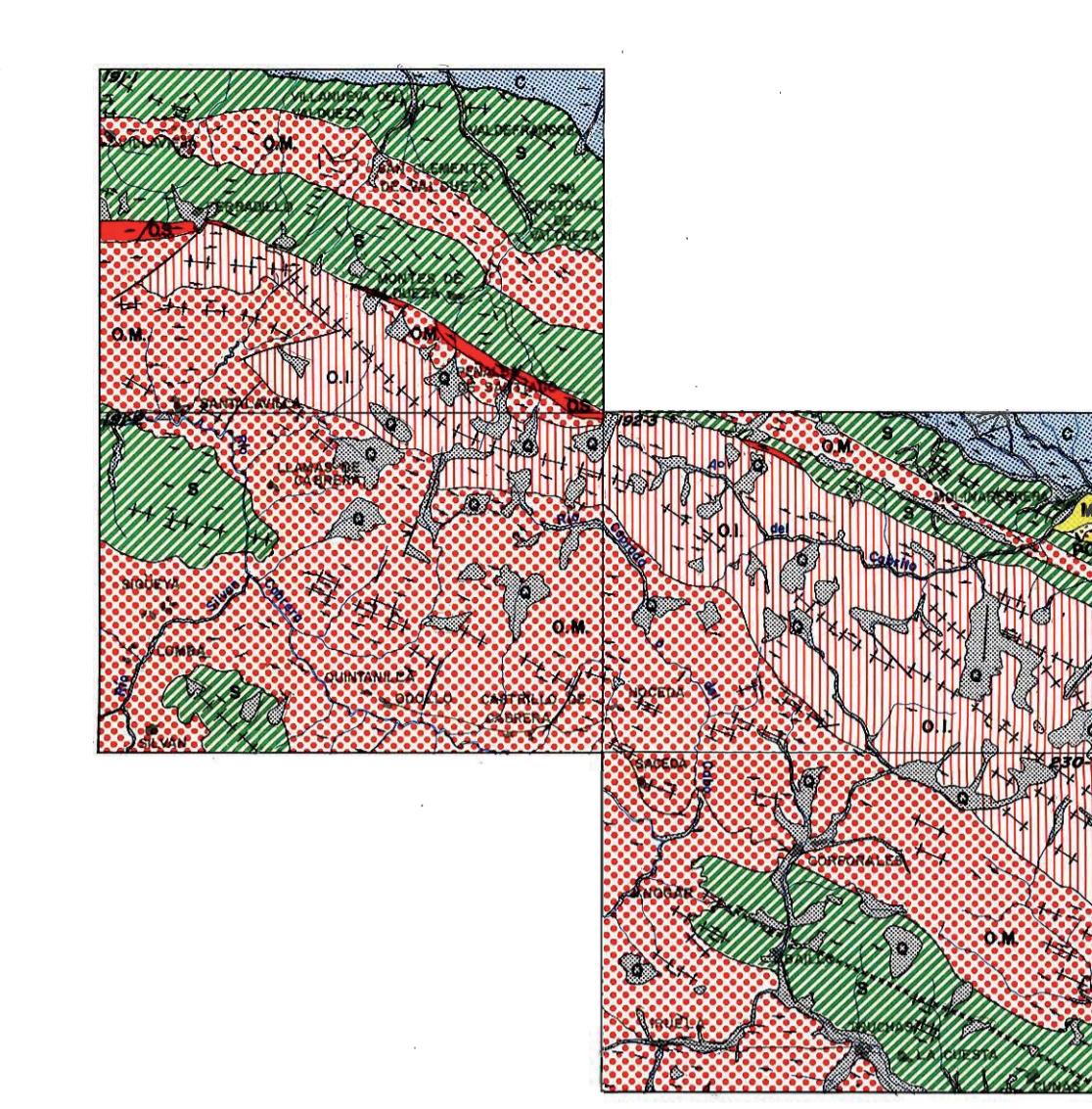
ESQUEMA GEOLOGICO / ESCALA 1: 200.000
