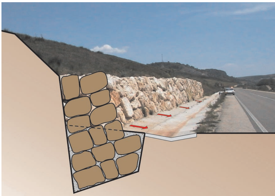
FIGURA 2.3. HORMIGÓN DE CIMENTACIÓN DE UN MURO DE ESCOLLERA CON PENDIENTE VERTIENTE HACIA LA CUNETETA DE PIE.
