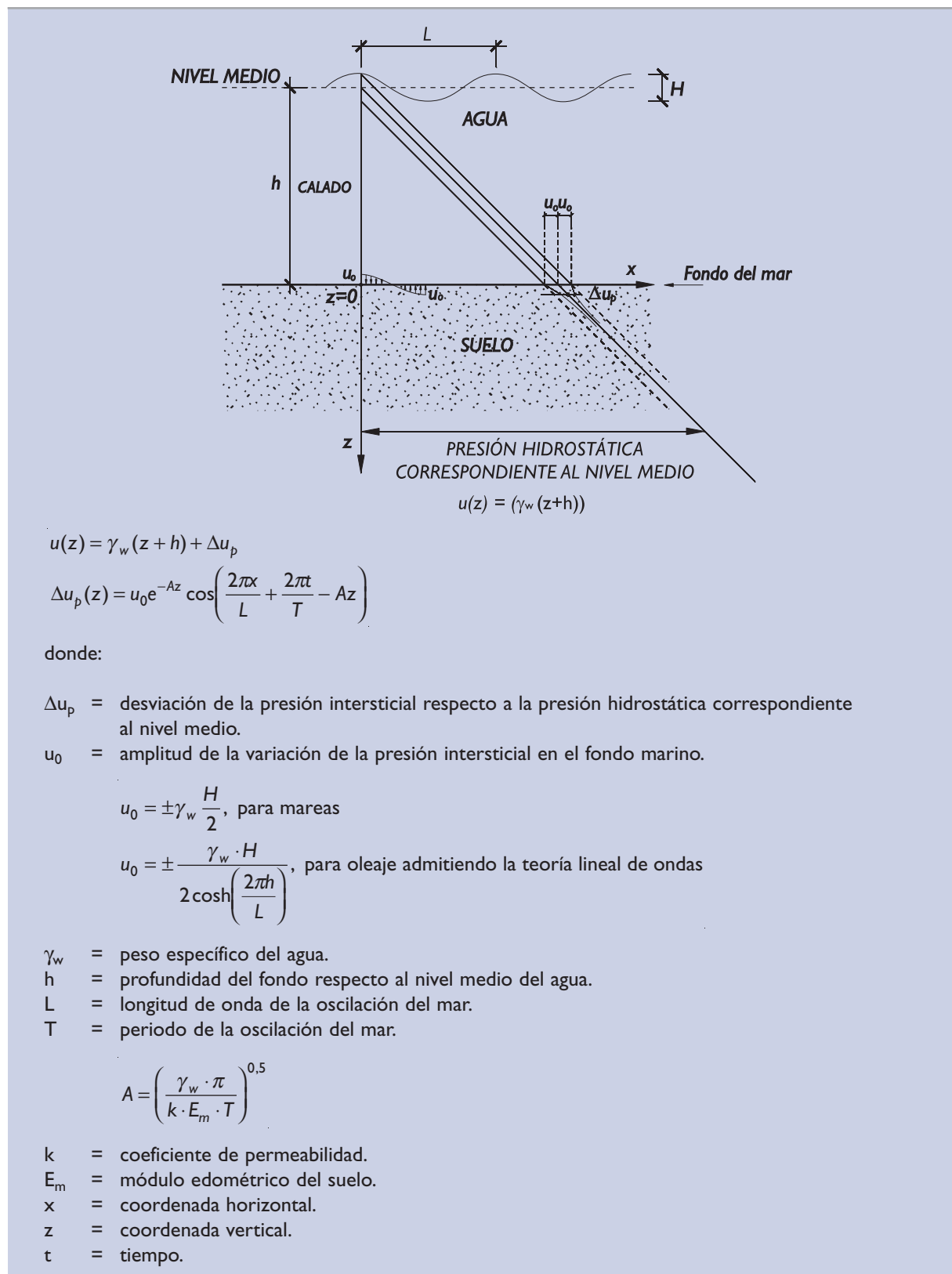
Figura 3.4.10. Estimación de la variación en la Ley de Presiones Intersticiales del fondo marino para situación drenada bajo la acción del oleaje u otras oscilaciones del mar (de Rouck, 1991)*
