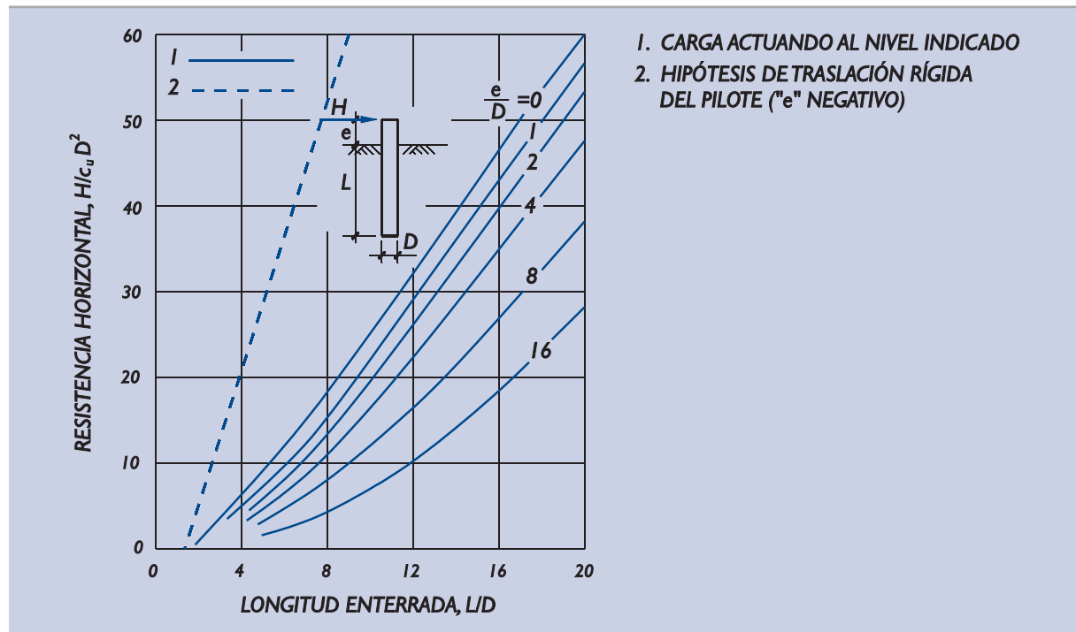
Figura 3.6.14. Rotura horizontal del terreno: suelos puramente cohesivos (Broms)
