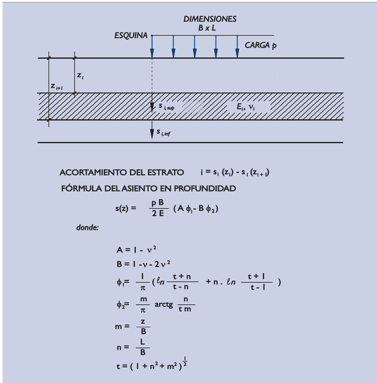
Figura 3.5.10. Fórmulas del método de Steinbrenner
