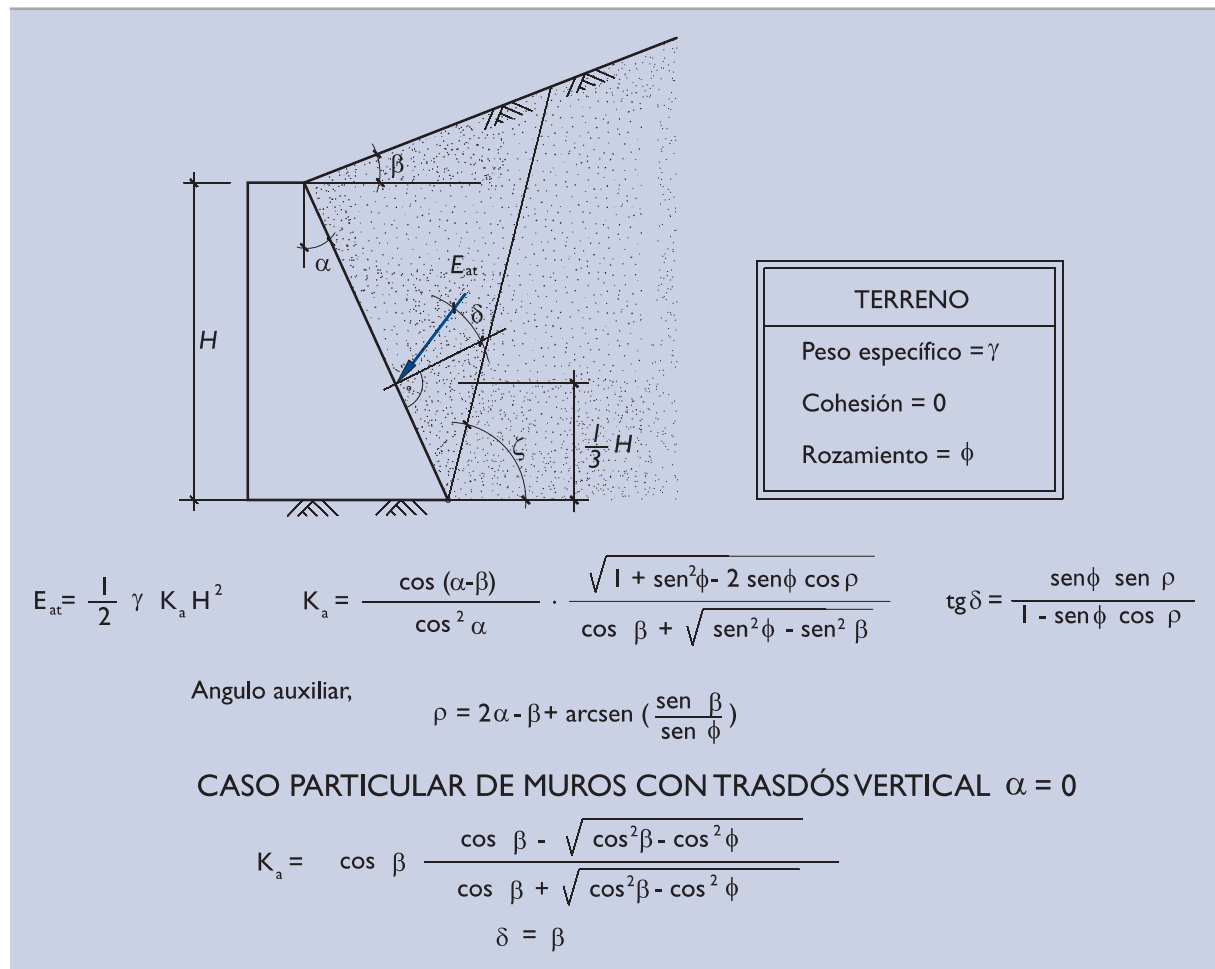
Figura 3.7.13. Geometría y solución del problema resuelto por Rankine
