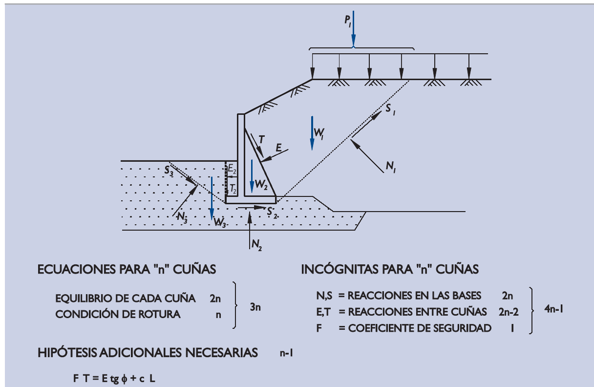
Figura 3.8.9. Esquema del método de las cuñas
