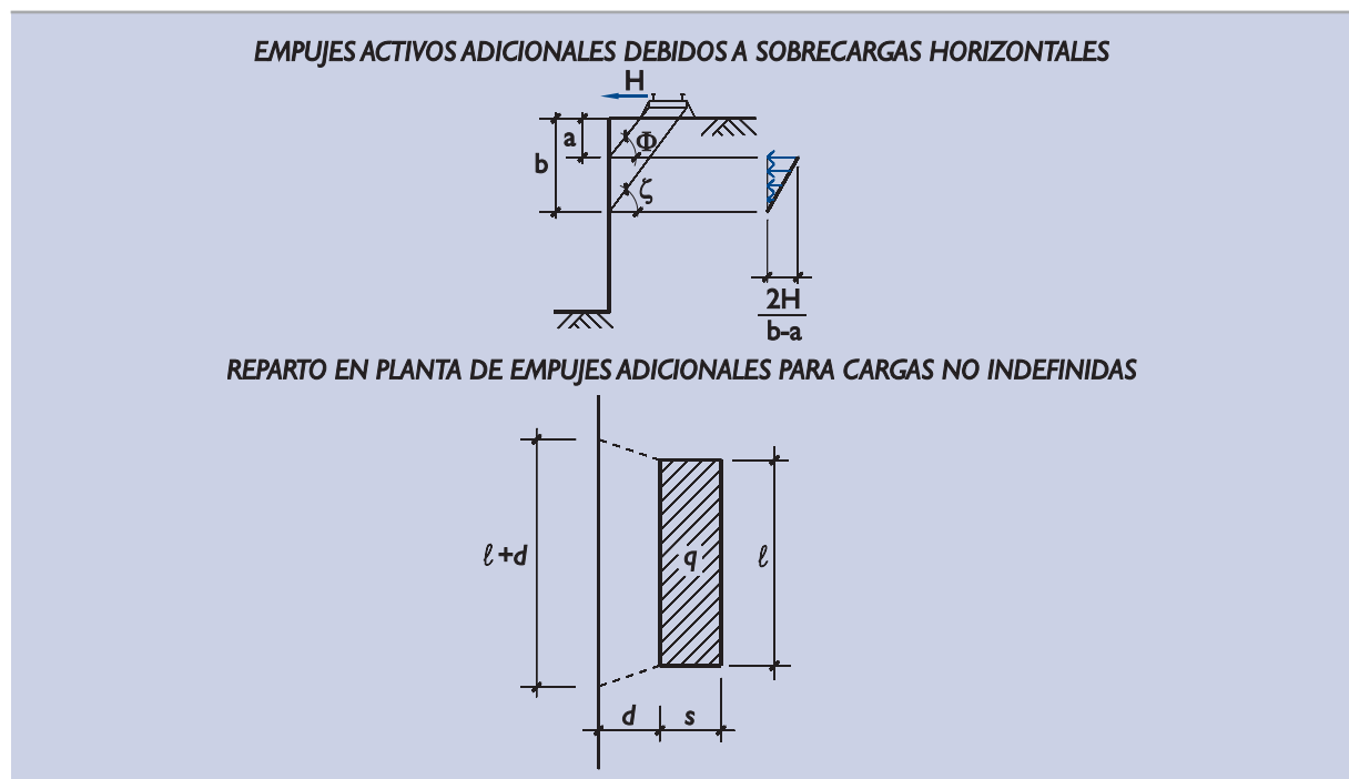
Figura 3.7.20. Efectos de otras sobrecargas
