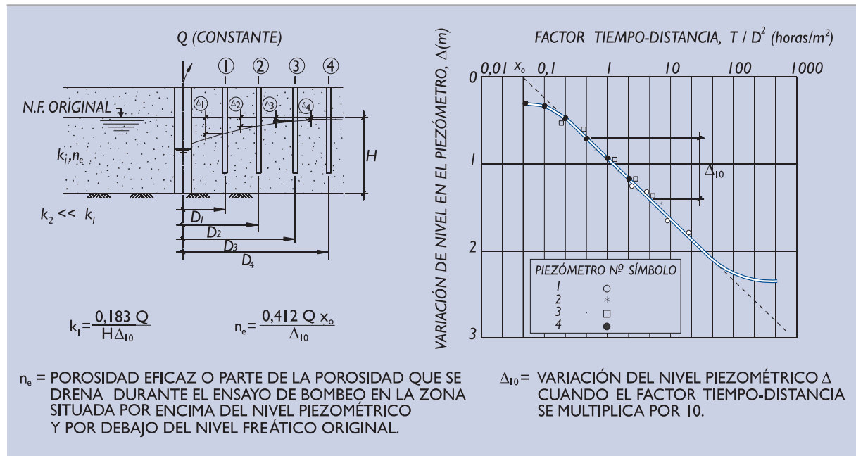
Figura A1.3. Esquema del ensayo de bombeo en régimen transitorio
