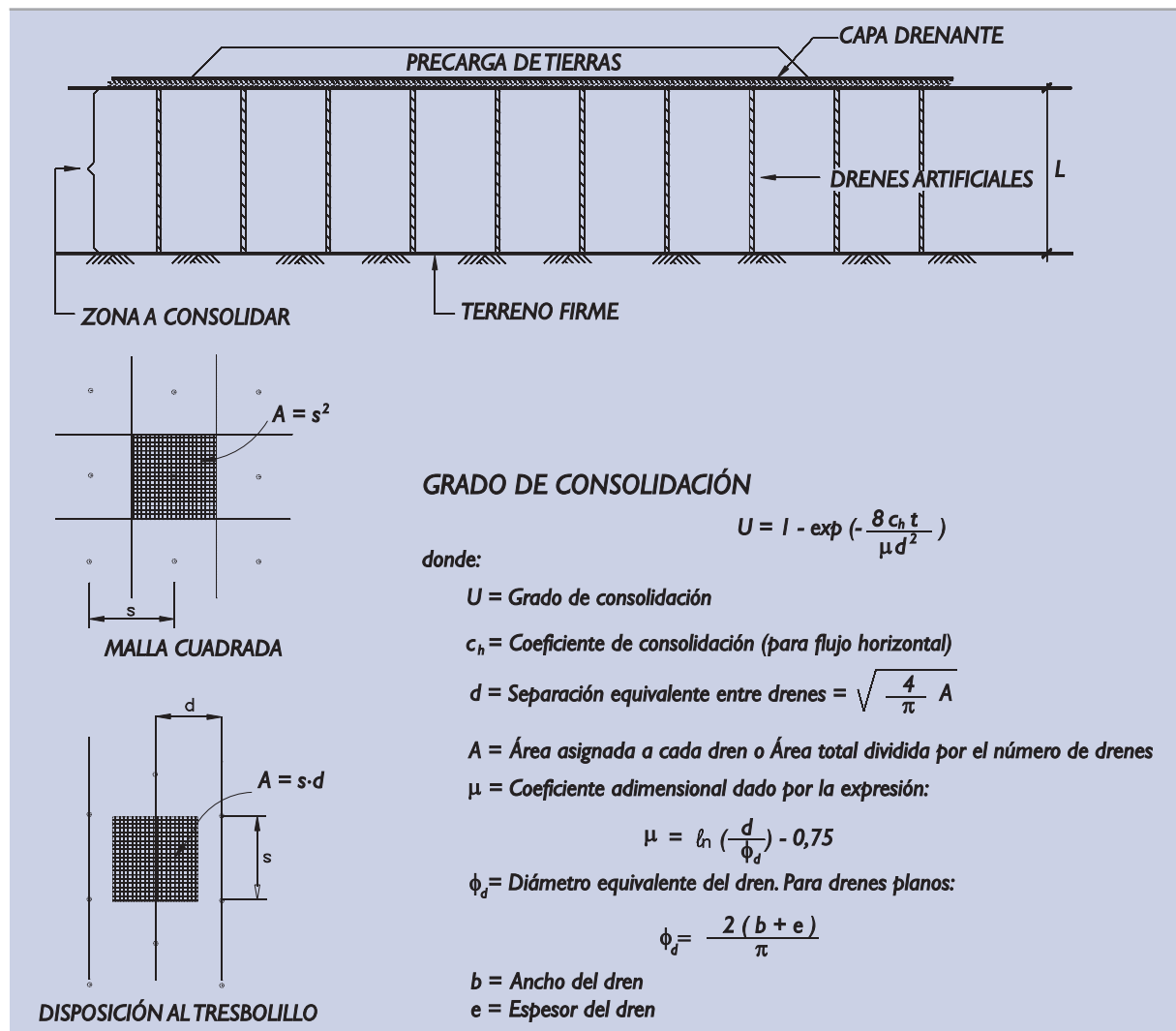
Figura 3.9.1. Estimación del grado de consolidación de precargas con drenaje acelerado
