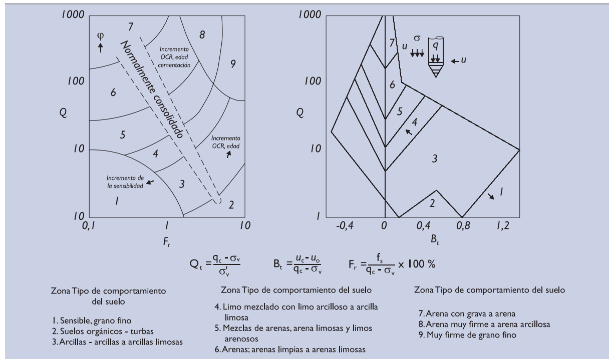
Figura 2.9.5. Clasificación del suelo a partir de los resultados del piezocono CPTU
