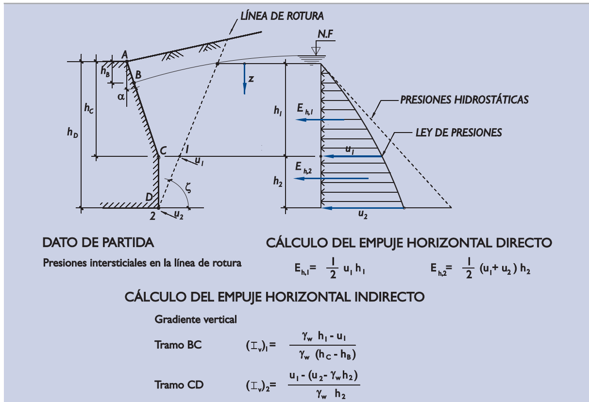
Figura 3.7.15. Cálculo del empuje horizontal del agua
