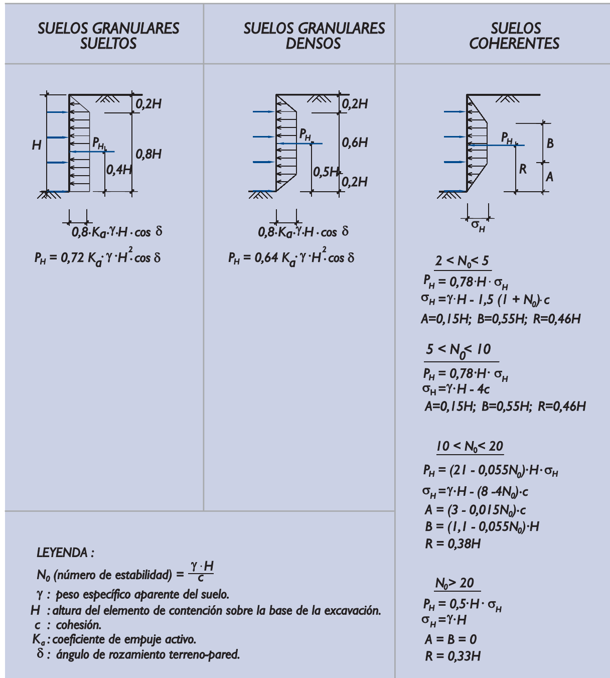
Figura 3.7.31. Empujes del terreno sobre entibaciones
