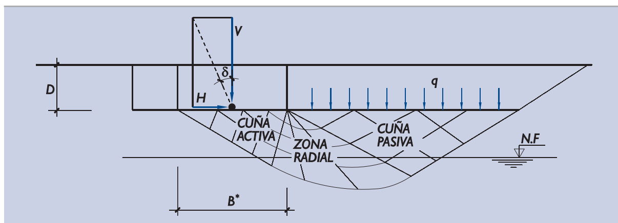
Figura 3.5.4. Geometría del posible hundimiento
