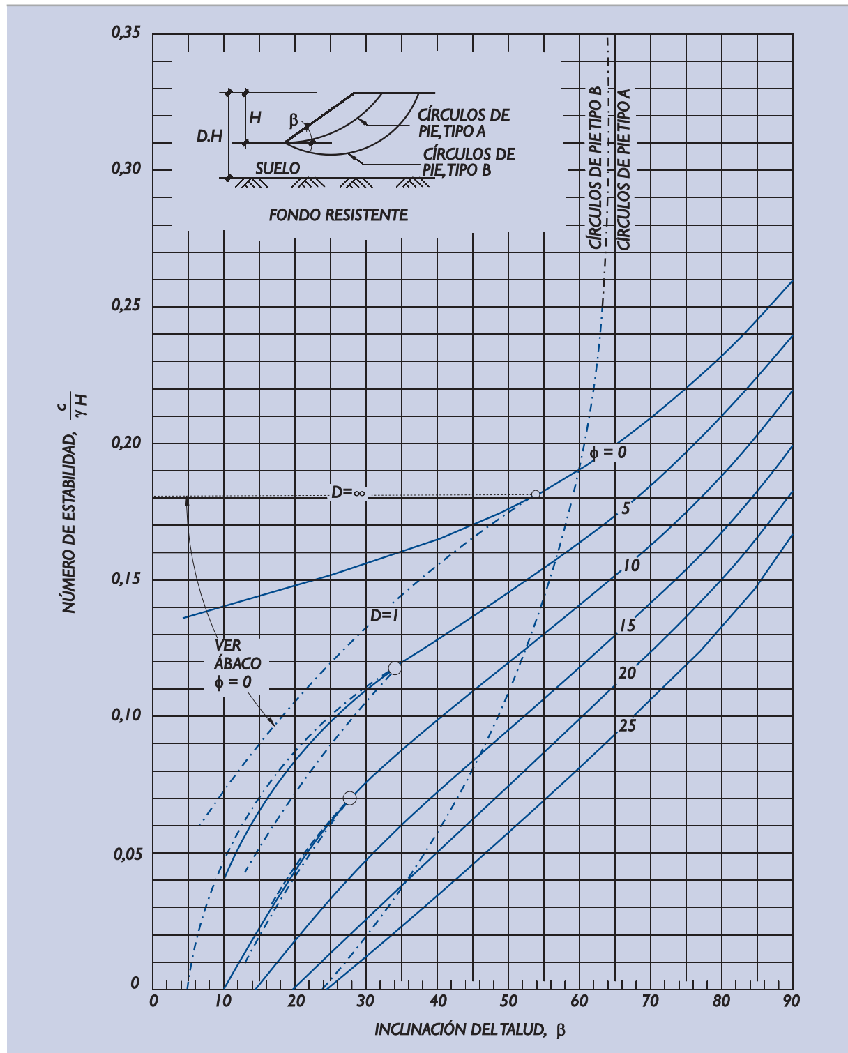
Figura 3.8.6. Ábaco de Taylor. Caso general, \phi \neq 0
