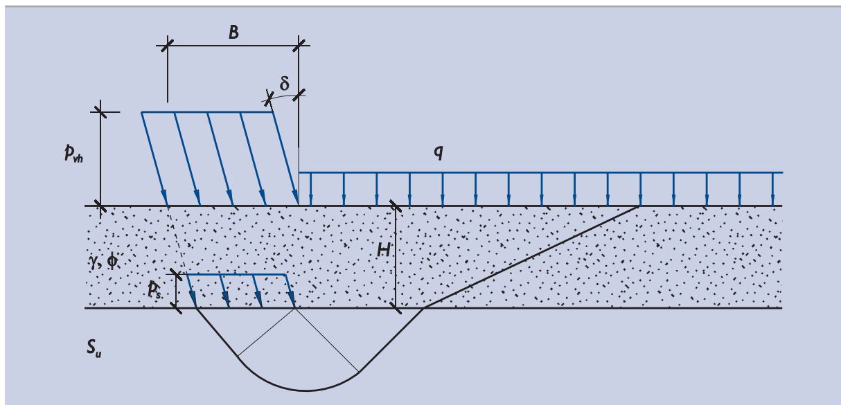
Figura 3.5.7. Esquema de la rotura de una banqueta granular apoyada sobre un suelo blando sin drenaje
