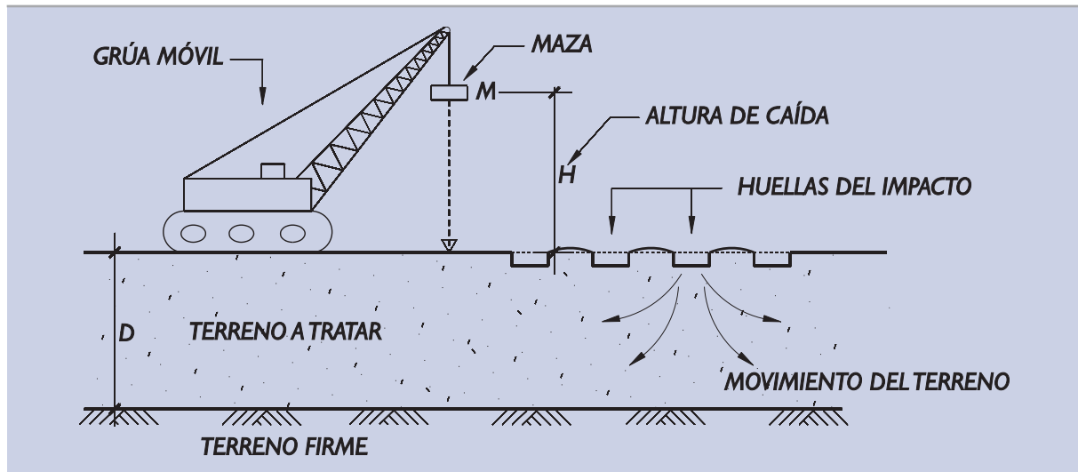
Figura 3.9.3. Esquema de la compactación dinámica
