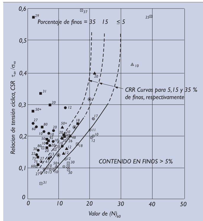
Figura 3.10.7. Resistencia a la licuefacción (20)
