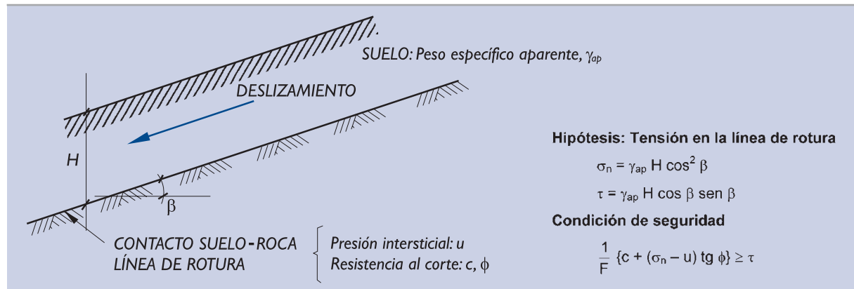
Figura 3.8.3. Comprobación de seguridad frente al deslizamiento plano indefinido
