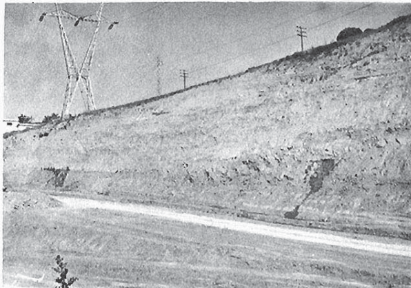
Foto 3-34 — Rezume de agua a través de un nivel arenoso en un talud sobre el grupo 32a (vista general y detalle).
