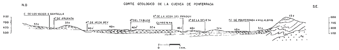
Fig. 3-15 — 40n' - Aluvial de gravas y arenas. — 40n - Terraza de gravaa y arenas. 32a - Arcillas y limos arenosos. — 12d - Pizarras grises con andalucita. — Pg - Granito de grano grueso.
