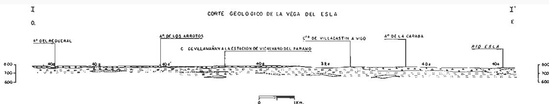
Fig. 3-5 – 40a - Aluvial de gravas, arenas y finos. – 40e - Terrazas de gravas y arenas cuarcíticas. 40d' - Aluvial de gravas, arenas y finos. – 40g - Gravas y arenas con matriz limo-arcillosa. – 32a - Arcillas y limos arenosos.
