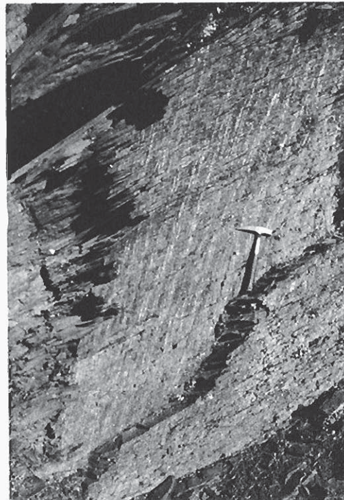
Foto 3-14 — Esquistosidad de fractura en pizarras Ordovícicas.
