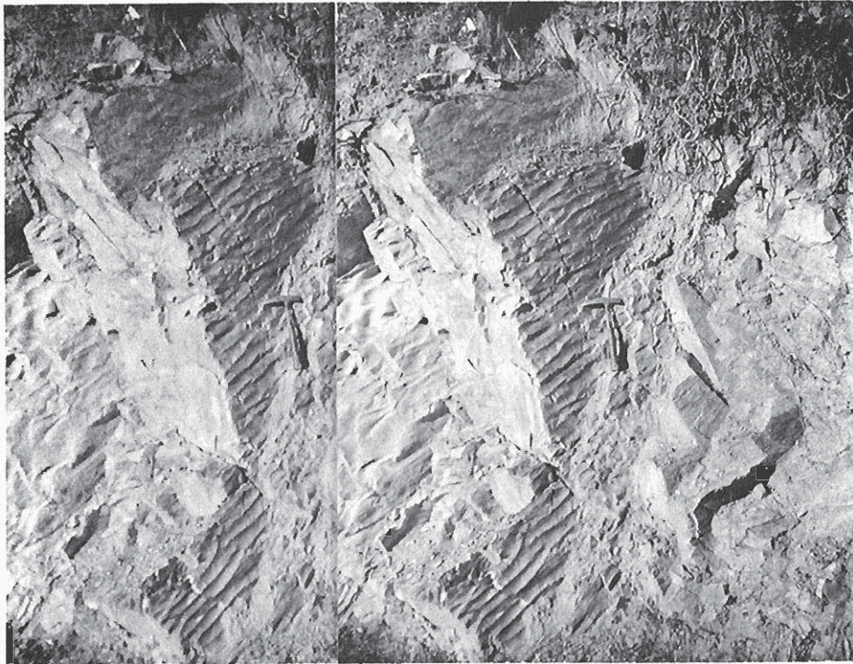
Foto 3-16 — Aspecto estéreo de cuarcitas y pizarras Ordovícicas.
