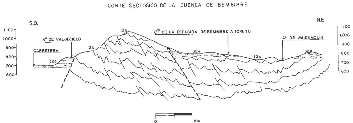
Fig. 3-16 — 32a - Arcillas y limos arenosos. — 13c - Pizarras y cuarcitas. 13b - Cuarcitas y pizarras. — 12b - Pizarras grises.
