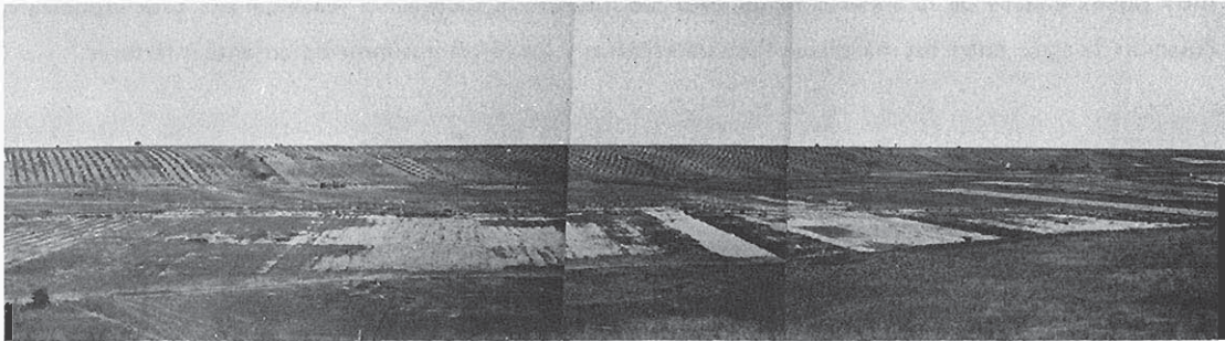
Foto 3-7 — Aspecto del encharcamiento que en pleno estío existe dentro de las zonas endorreicas.
