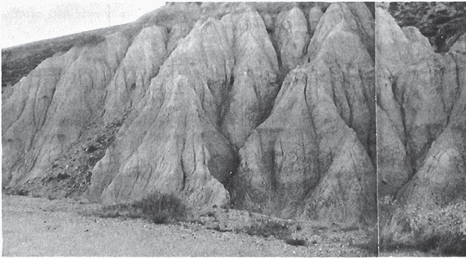
Foto 3-2 — Arcillas arenosas del grupo (32a)
