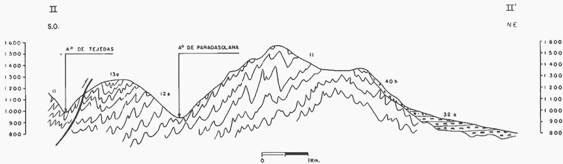
Fig. 3-12 — 40h - Coluvial de cantos de cuarcita.
