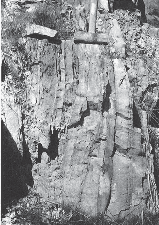
Foto 3-20 — Micropliegues de arrastre de las capas del grupo (11).
