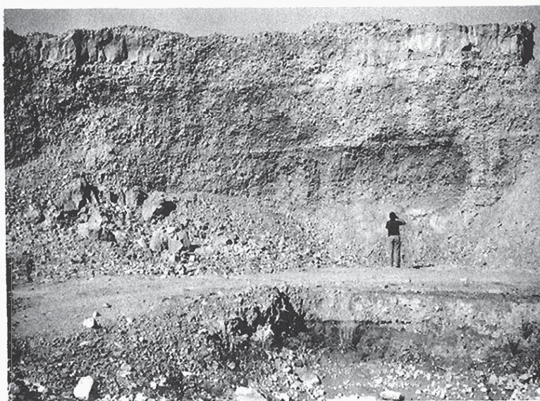
Foto 3-39 — Terraza de ocho metros de potencia. (40n).
