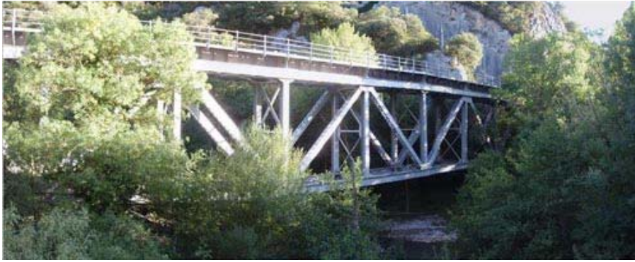
Ilustración 8. Celosía Warren en Trespaderne, Burgos. La vegetación tapa una visión completa del puente, 90 años después de su entrada en servicio
