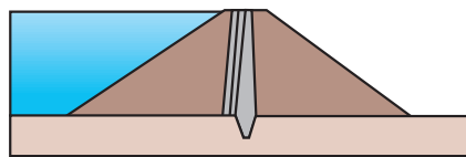
Azud de escollera
