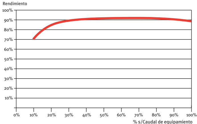
Rendimiento turbina Pelton
