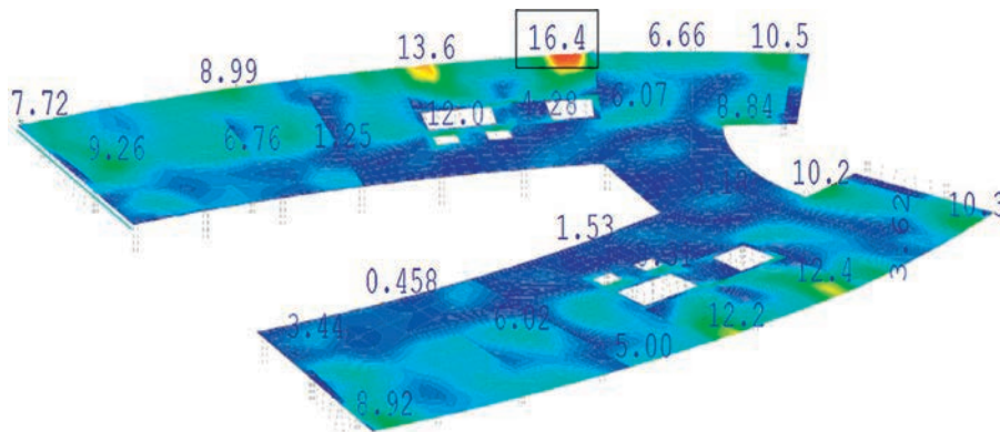
Figura 15. Momentos torsores (kN·m/m) en losas debidos a la acción sísmica. SEMPLANTA +2.
