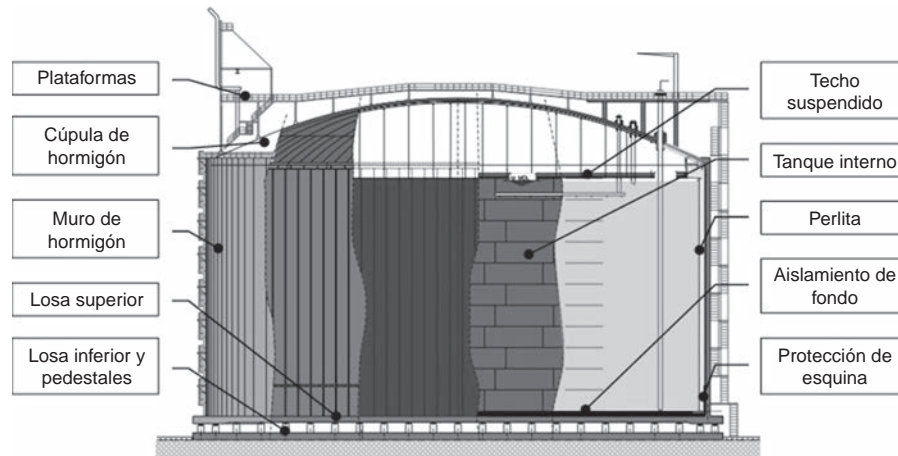
Figura 3. Esquema de tanque de GNL, tipo contención total, sobre aisladores sísmicos.
