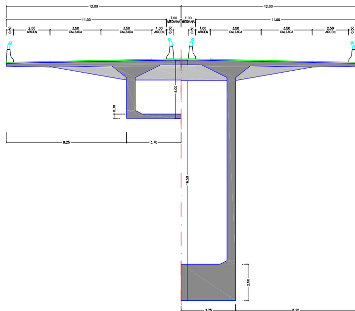
Figura 13. Solución propuesta. Sección transversal por centro de vano y apoyos
